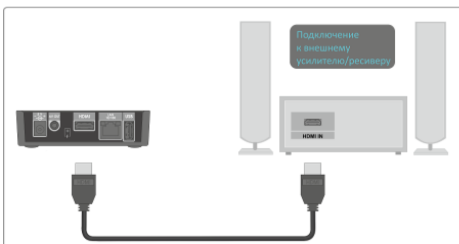
Рисунок 14 – Подключение медиацентра к акустической системе с разъемом HDMI
