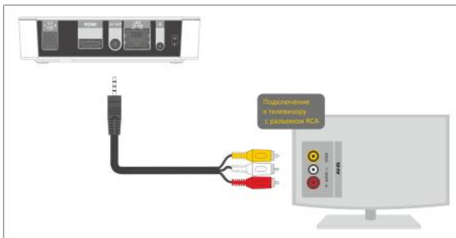
Рисунок 8 – Подключение к телевизору по интерфейсу RCA
