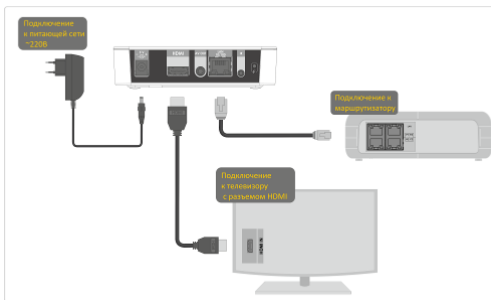
Рисунок 11 – Пример подключения медиацентра NV-300
