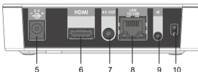
Рисунок 3 – Внешний вид задней панели STB NV-300
