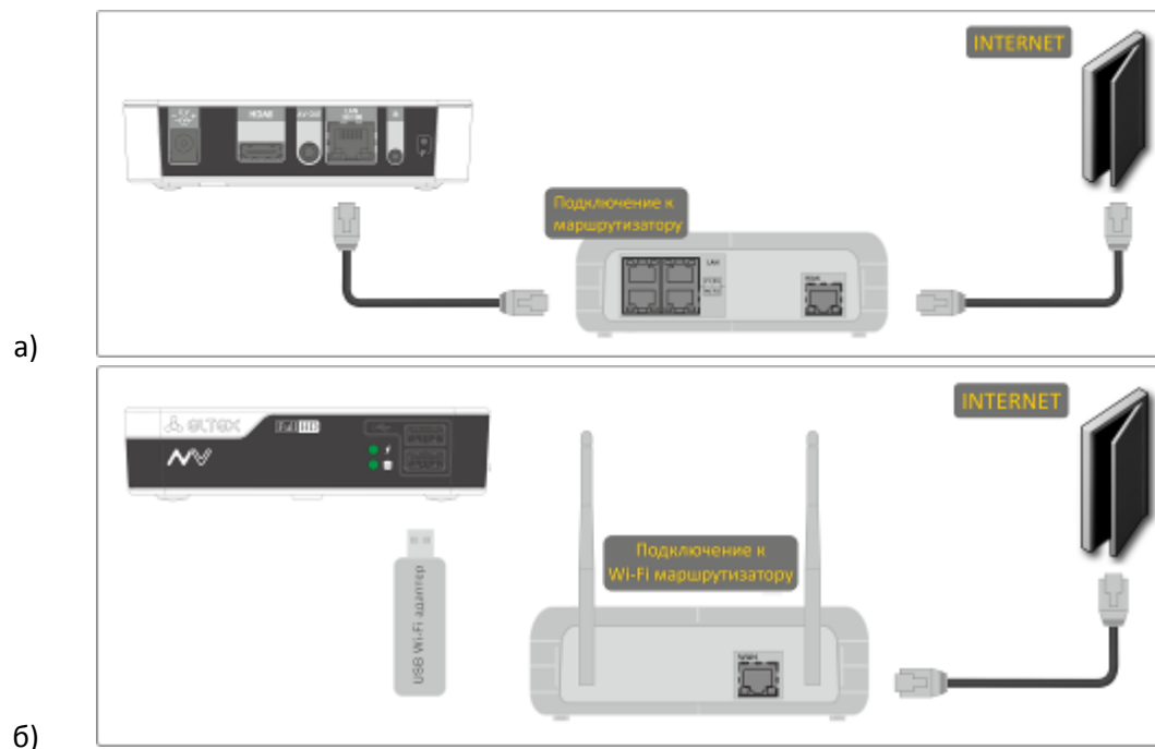
Рисунок 10 – Подключение к сети провайдера, используя маршрутизатор
