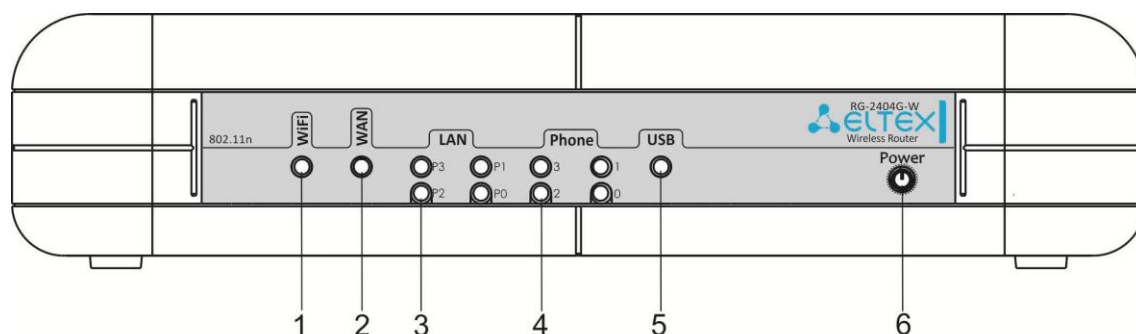
Рисунок 4 – Внешний вид передней панели RG-2404G-W
