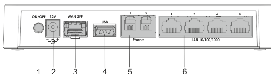
Рисунок 7 – Внешний вид задней панели RG-4402GF-W
