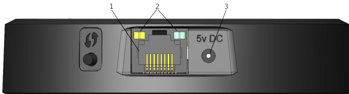
Рисунок 3 — Внешний вид задней панели WEP-1L
