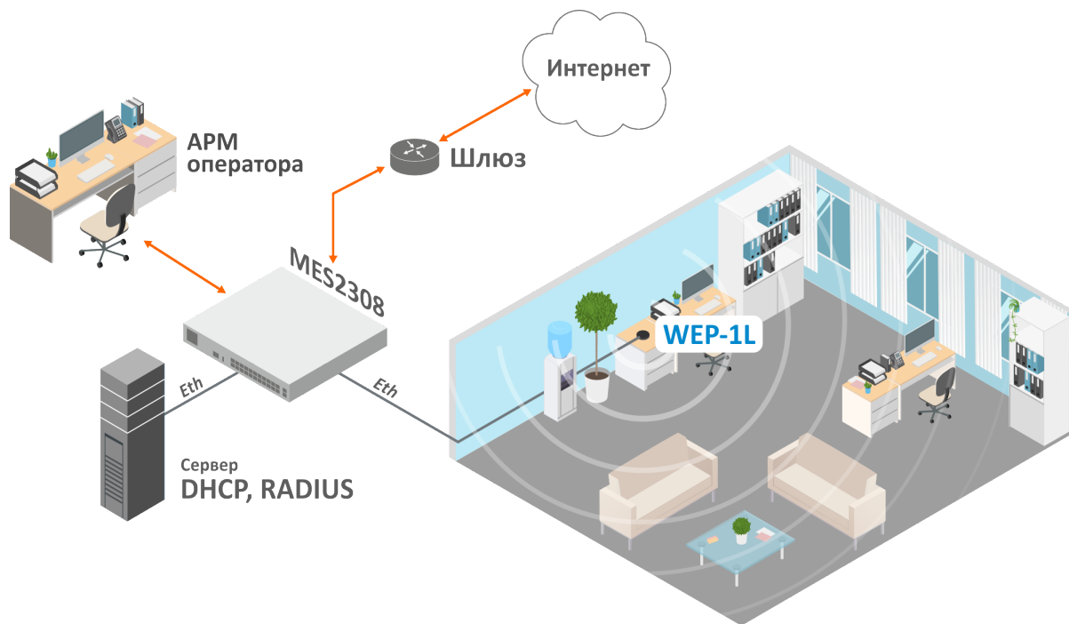
Рисунок 1 — Функциональная схема использования WEP-1L
