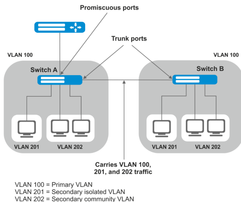
Рисунок 53 — Пример работы технологии Private VLAN
