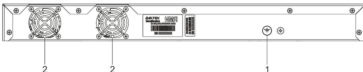
Рисунок 32 — Задняя панель MES2324P ACW
