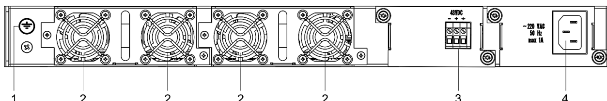
Рисунок 25 — Задняя панель MES5324
