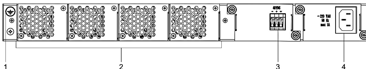
Рисунок 28 — Задняя панель MES3324F, MES3348F, MES3324
