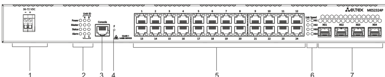
Рисунок 9 — Передняя панель MES2324P DC
