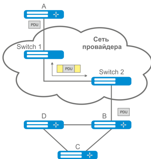
Рисунок 54 — Пример работы функции L2PT
