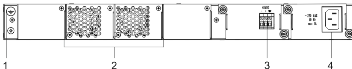
Рисунок 26 — Задняя панель MES3308F
