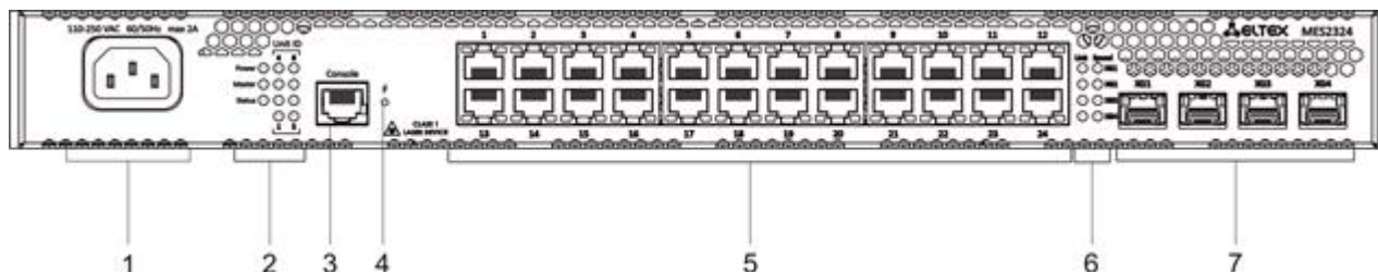
Рисунок 6 — Передняя панель MES2324 AC
