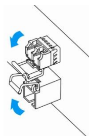
Рисунок 51 — Открытие защелки SFP-трансиверов
