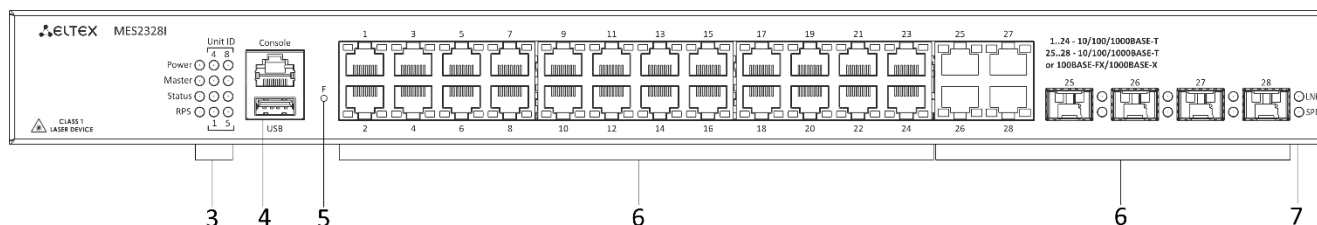
Рисунок 15 — Передняя панель MES2328I
