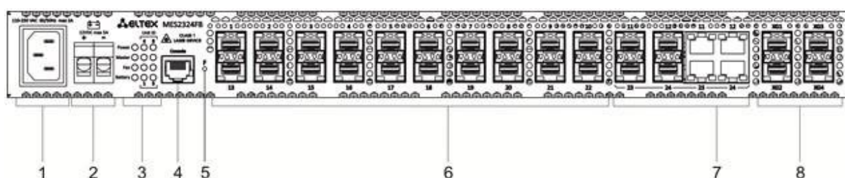
Рисунок 12 — Передняя панель MES2324FB
