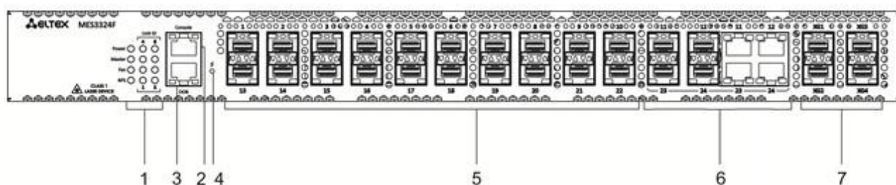
Рисунок 2 — Передняя панель MES3324F
