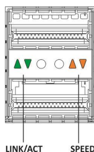
Рисунок 41 — Внешний вид разъема с QSFP+-трансиверами
