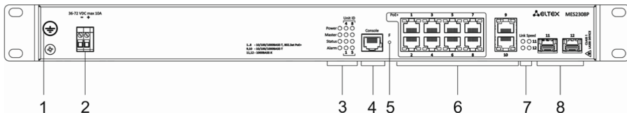
Рисунок 20 — Передняя панель MES2308P DC
