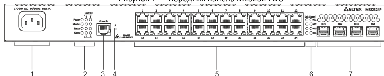
Рисунок 8 — Передняя панель MES2324P AC, MES2324P ACW
