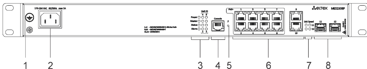
Рисунок 19 — Передняя панель MES2308P AC
