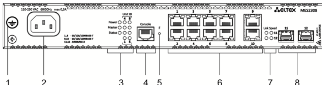
Рисунок 18 — Передняя панель MES2308
