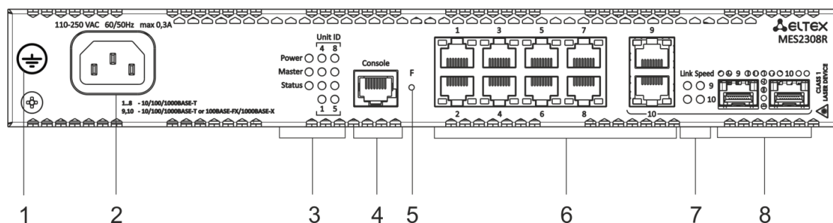
Рисунок 21 — Передняя панель MES2308R
