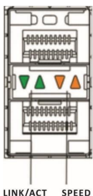
Рисунок 42 — Внешний вид разъема SFP/SFP+
