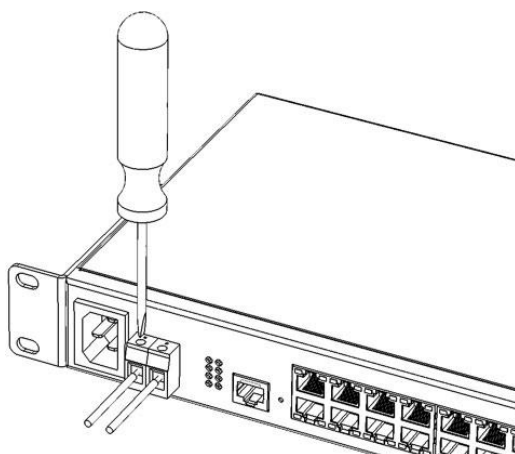
Рисунок 48 — Подключение АКБ к устройству
