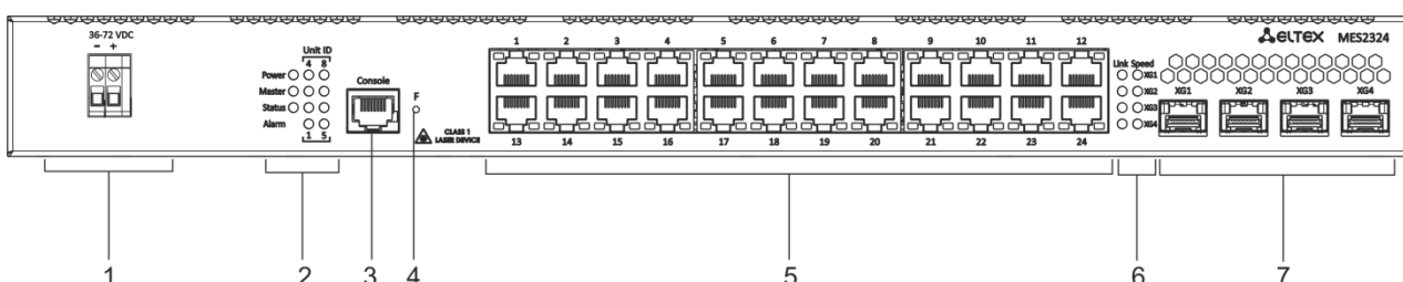
Рисунок 7 — Передняя панель MES2324 DC
