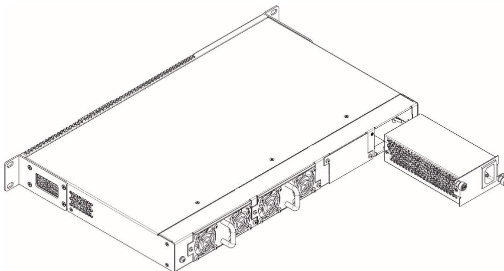
Рисунок 47 — Установка модулей питания
