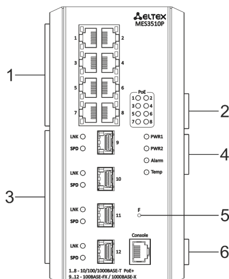
Рисунок 24 — Передняя панель MES3510P
