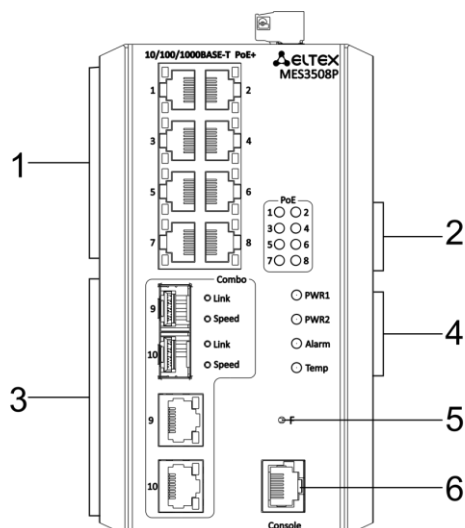
Рисунок 23 — Передняя панель MES3508P
