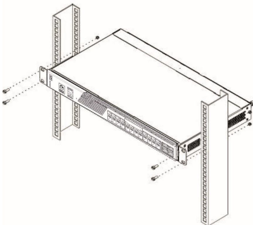
Рисунок 45 — Установка устройства в стойку
