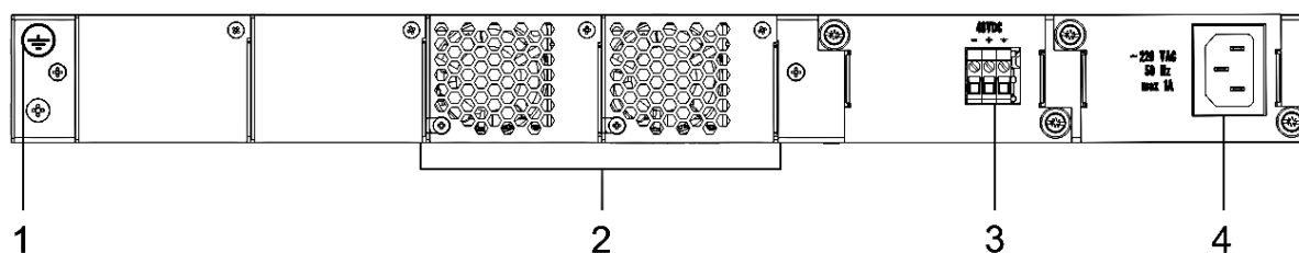
Рисунок 29 — Задняя панель MES3348
