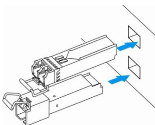
Рисунок 49 — Установка SFP-трансиверов
