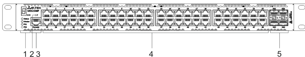
Рисунок 10 — Передняя панель MES2348P
