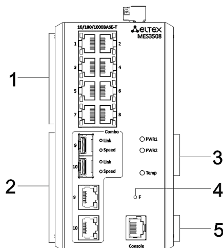
Рисунок 22 — Передняя панель MES3508
