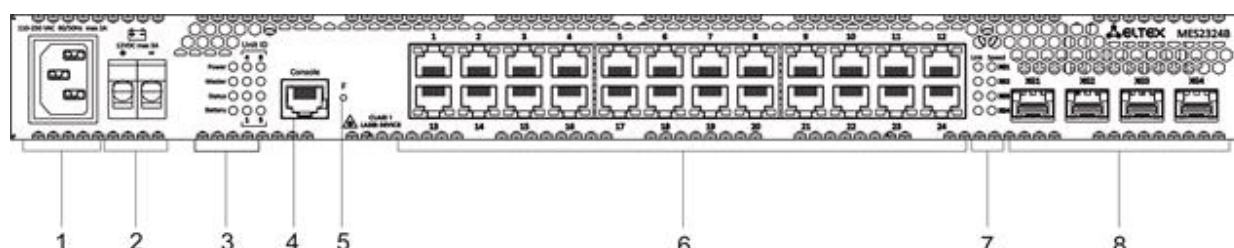
Рисунок 11 — Передняя панель MES2324B
