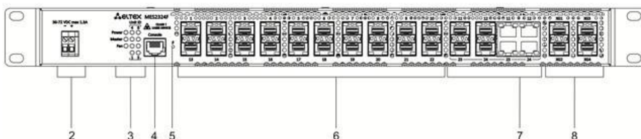
Рисунок 13 — Передняя панель MES2324F DC
