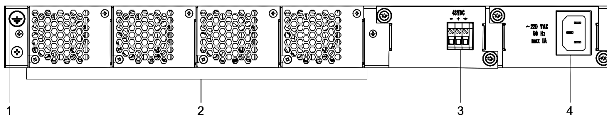
Рисунок 24 — Задняя панель MES3324F, MES3348F, MES3324
