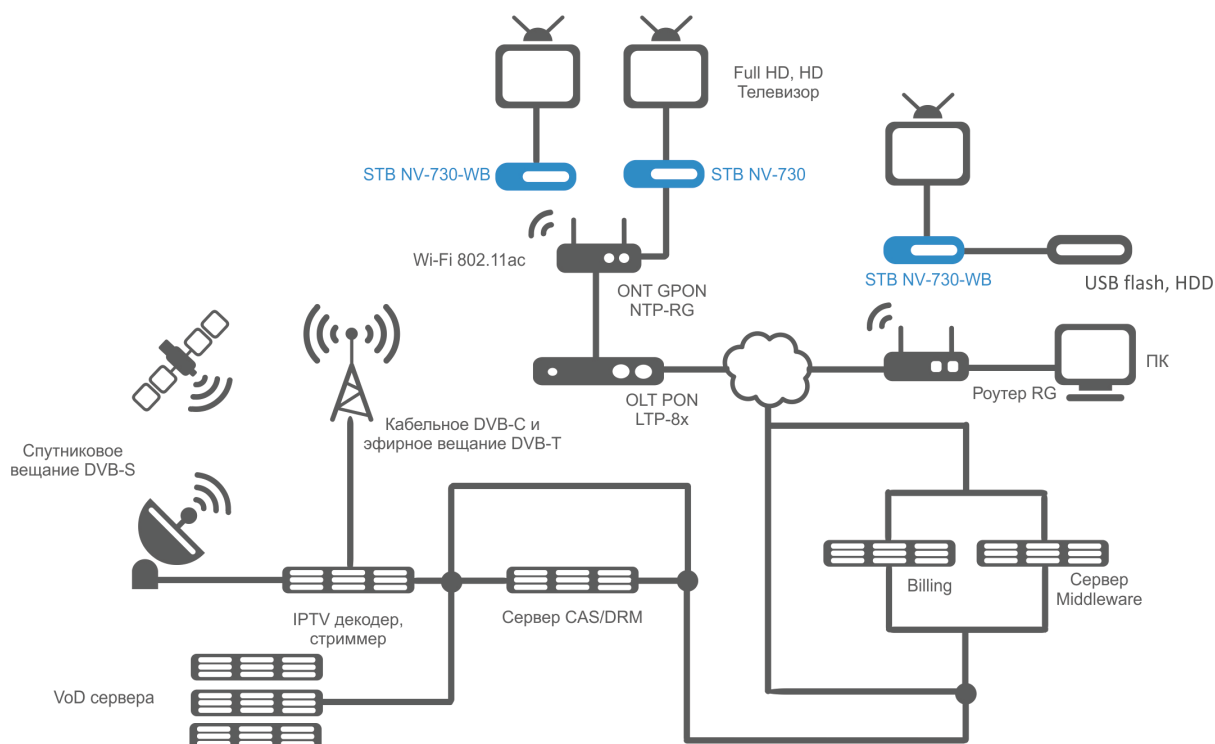
Рисунок 1 — Схема применения
