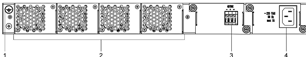
Рисунок 22 — Задняя панель MES3324F, MES3348F, MES3324
