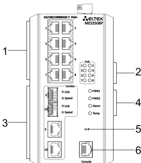
Рисунок 19 — Передняя панель MES3508P
