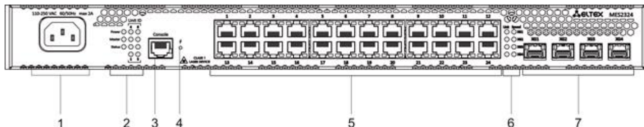
Рисунок 6 — Передняя панель MES2324
