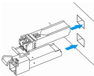
Рисунок 42 — Установка SFP-трансиверов
