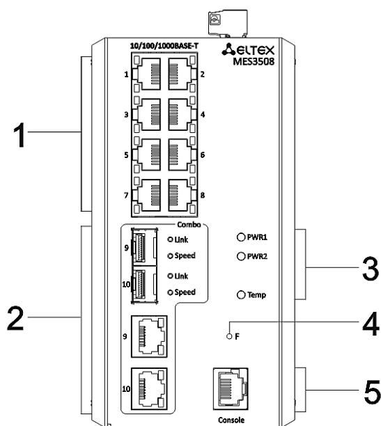
Рисунок 20 — Передняя панель MES3508
