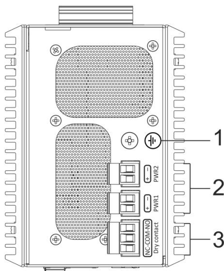
Рисунок 31 — Верхняя панель MES3508 и MES3508P
