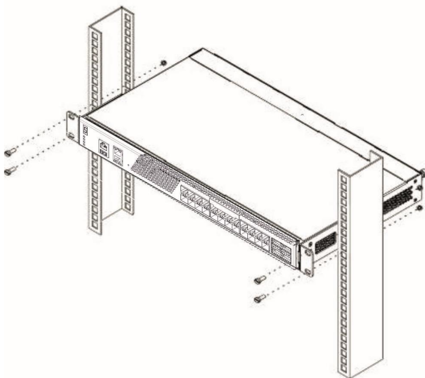
Рисунок 38 — Установка устройства в стойку
