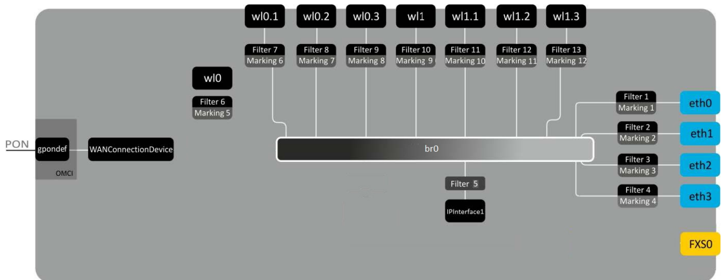
Рисунок 14 – Логическая архитектура устройства с заводской конфигурацией
