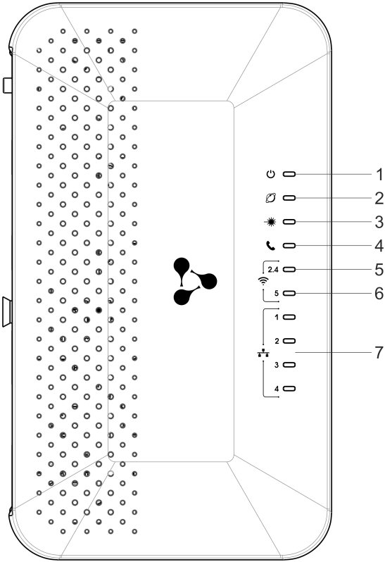
Рисунок 13 – Внешний вид верхней панели NTU-RG-5421G-Wac rev.B и NTU-RG-5421G-WZ rev.B Текущее состояние устройства отображается при помощи индикаторов, расположенных на верхней панели. Перечень состояний индикаторов приведен в таблице 11 . Таблица 11 – Описание индикаторов верхней панели NTU-RG-5421G-Wac rev.B, NTU-RG-5421G-WZ rev.B
