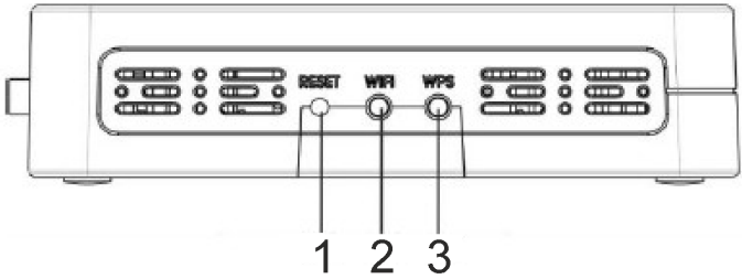
Рисунок 9 – Внешний вид боковой панели NTU-RG-5402G-W, NTU-RG-5421G-Wac и NTU-RG-5421G-WZ На боковой панели устройства расположены следующие кнопки, таблица 7 .
